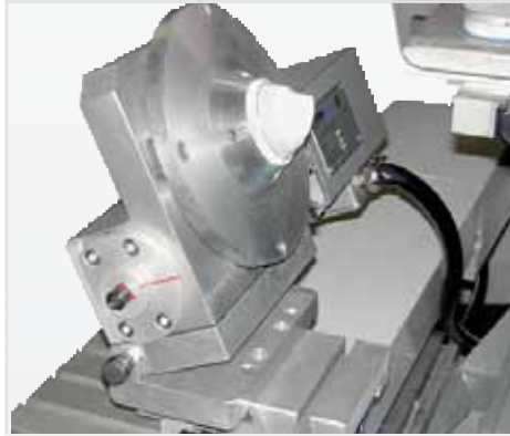
Tavola rotante TRCN 2.5 come 4° asse di rotazione su indexore PR 610 TRCN 2.5 rotary table working as 4° axes fixed on indexor PR 610
